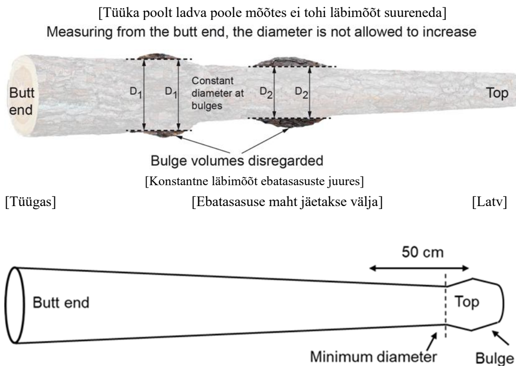
Joonis 4. Ebatasasuste korral läbimõõtu korrigeeritakse. Liikudes noti tüükapoolse otsa poolt ladvapoolse otsa poole ei tohi läbimõõt suureneda. Praktilistel põhjustel otsitakse vähimat läbimõõtu 50 cm ulatuses ebatasasuse kõige suuremast läbimõõdust alates.
