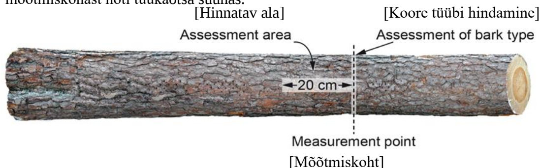
Joonis 6. Läbimõõdu automaatse mõõtmise korral hinnatakse koore tüüpi mõõtmiskohas. Koore maha hõõrdumist hinnatakse 0-20 cm ulatuses mõõtmiskohast noti tüükaotsa suunas.
