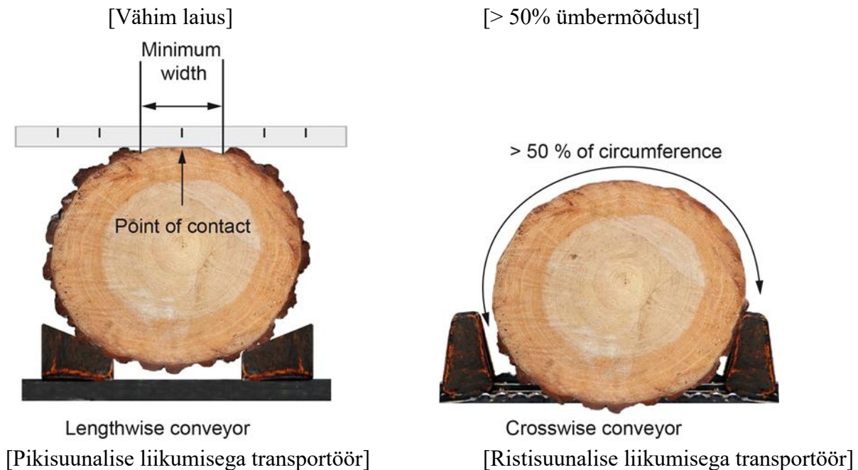
Joonis 8. Maha hõõrdunud koore hindamispõhimõtte pikisuunas liikaval transportööril, vasakul ja ristisuunas liikaval transportööril, paremal.
