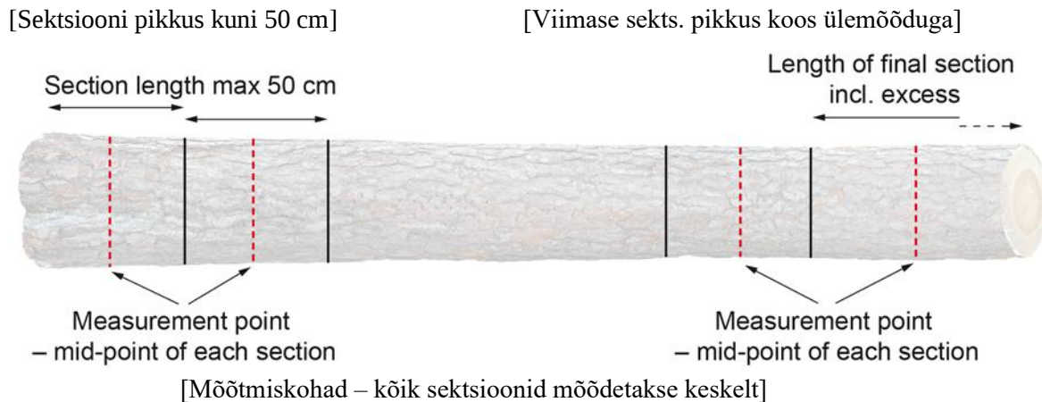
Joonis 13. Läbimõõdude mõõtmise kohad sektsiooniti mõõtmisel.
